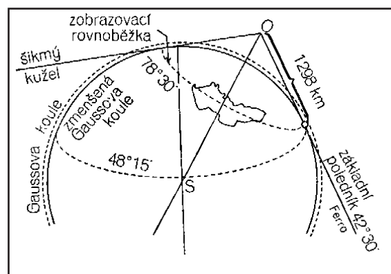
JTSK - Křovákovo zobrazení
