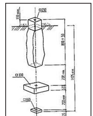
Stabilizace ZBPP JTSK
