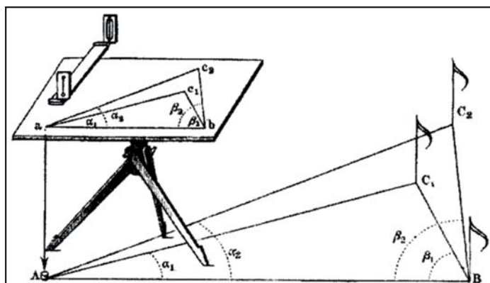
Obr. 2.2 d Měřický, topografický stolek a průzor s ukázkou protínání vpřed
