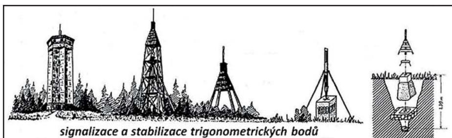
Obr. 2.2 c - signalizace bodů
